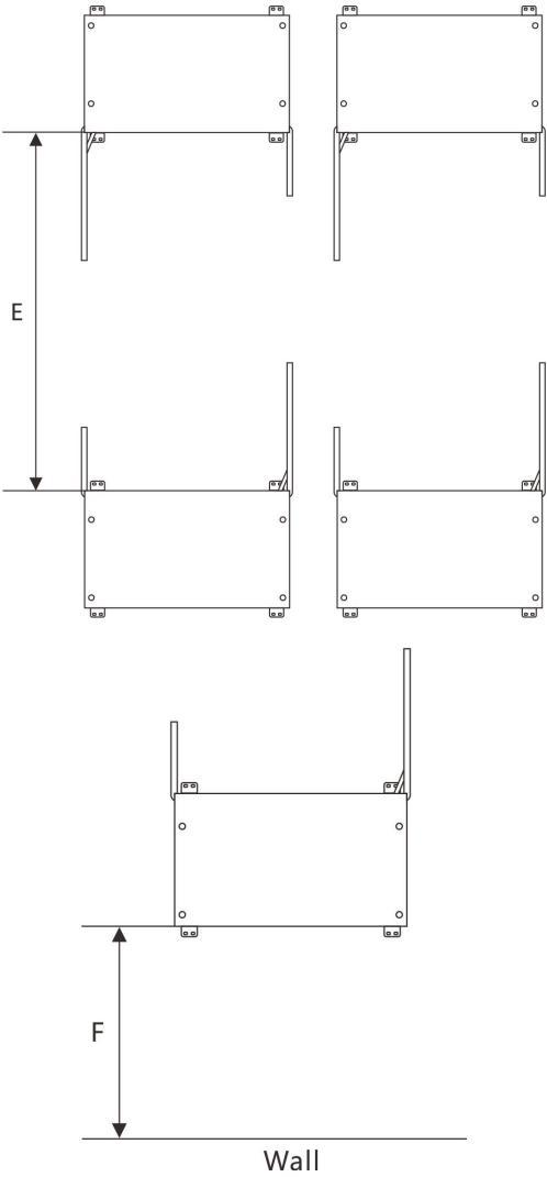
Zeichnung des Montagefreiraums (Draufsicht)
